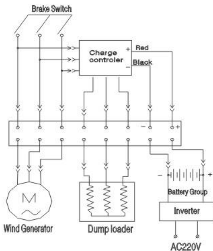
Рис. 8. Электрическая схема ветроэлектростанции
